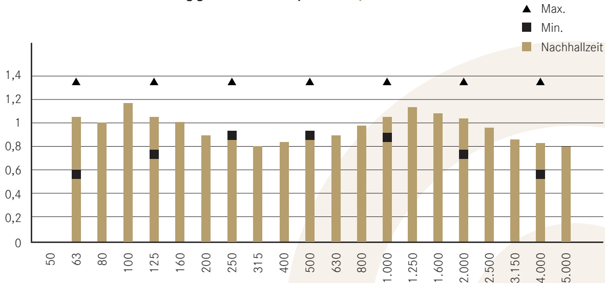
Diagramm - großer Saal: Bewertung lt. Toleranzbereich der optimalen Nachhallzeit nach ÖNORM B8115-3 in Abhängigkeit von der Frequenz für Sprache
