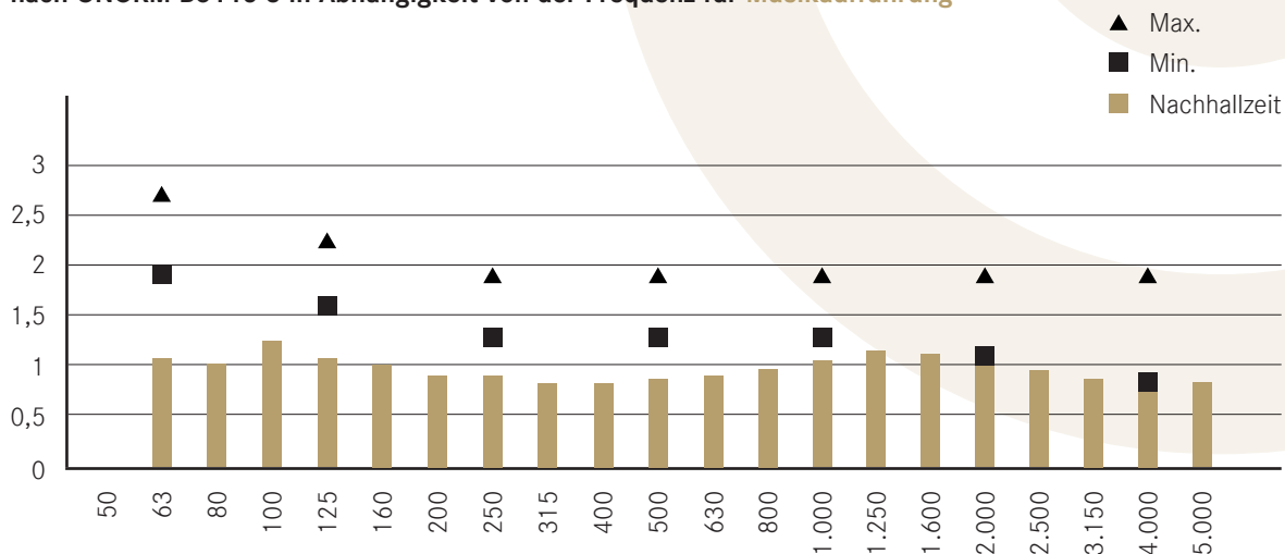
Diagramm - großer Saal: Bewertung lt. Toleranzbereich der optimalen Nachhallzeit nach ÖNORM B8115-3 in Abhängigkeit von der Frequenz für Musikaufführung
