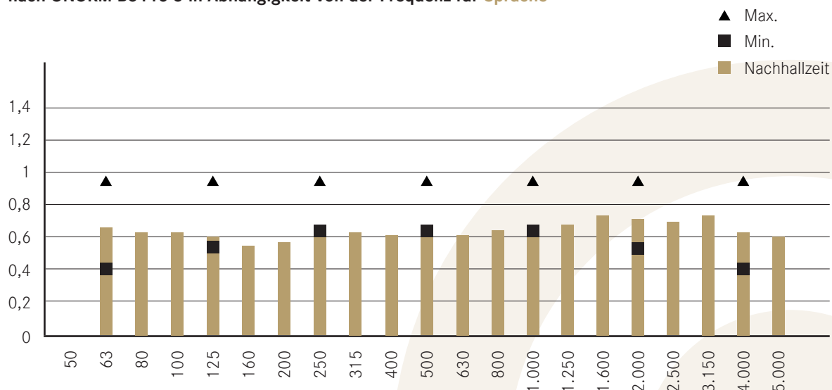
Diagramm - kleiner Saal: Bewertung lt. Toleranzbereich der optimalen Nachhallzeit nach ÖNORM B8115-3 in Abhängigkeit von der Frequenz für Sprache
